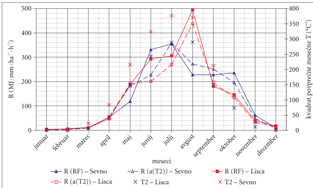
Slika 5: Primerjava erozivnosti dežja R, izračunane s programom RF in s pomočjo kvadratne enačbe a = a_0 + a_1 \cdot T^2 , ter kvadrata povprečnih mesečnih temperatur T za merilni mesti Lisca in Sevno.
